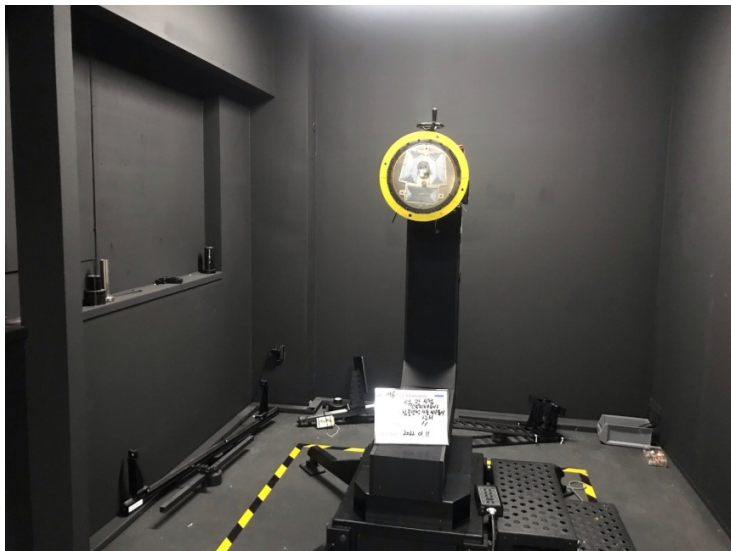
사진 1-1 시료 설치
