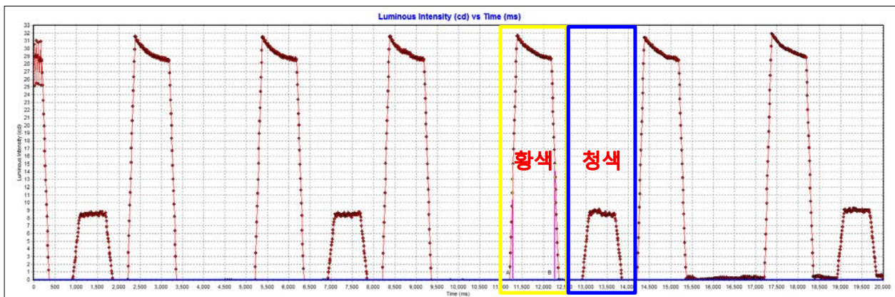
그림 1-1 시험결과(섬광 시험)
